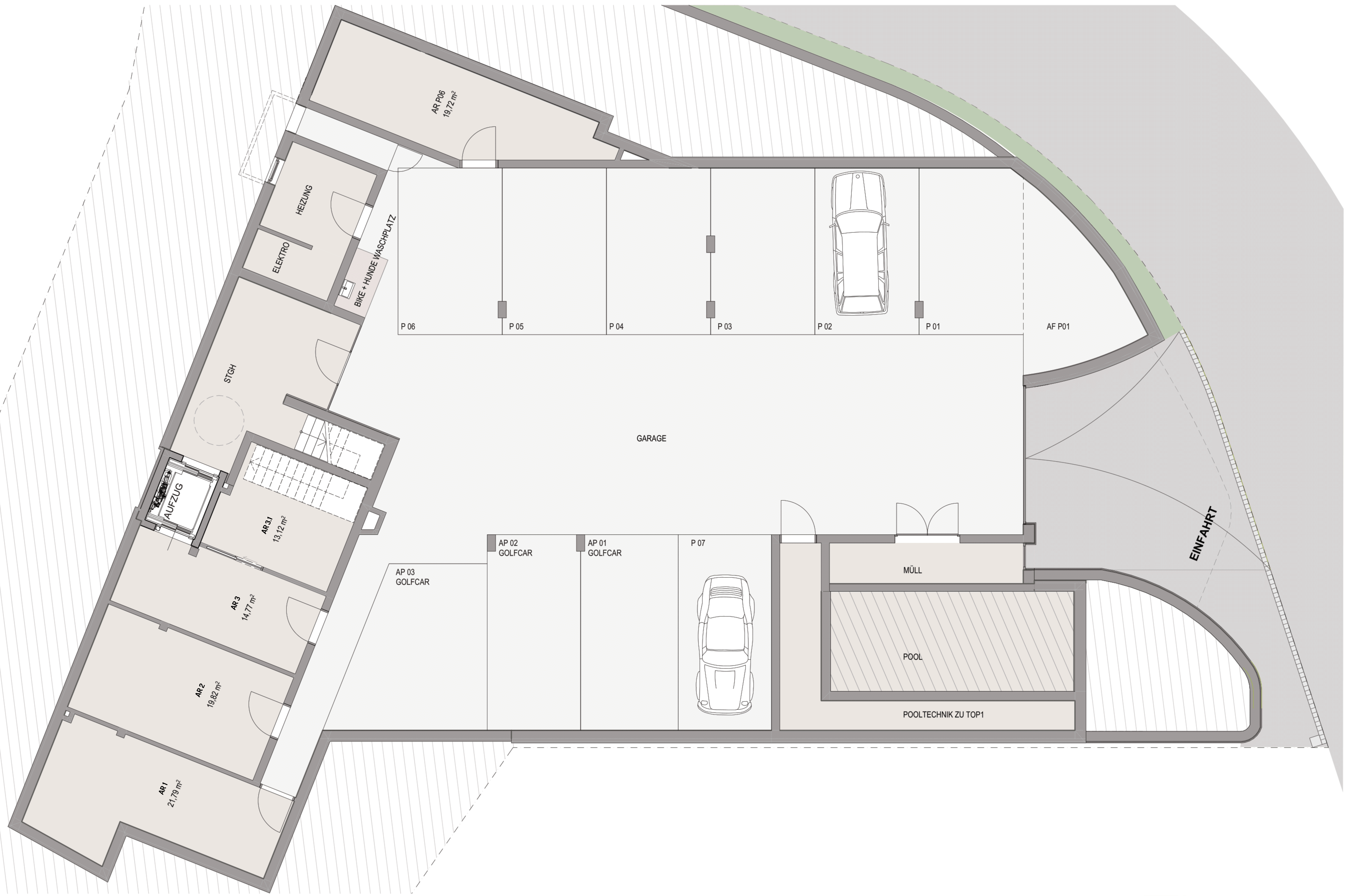
Garage / Keller - 1:100 06.06.2024
